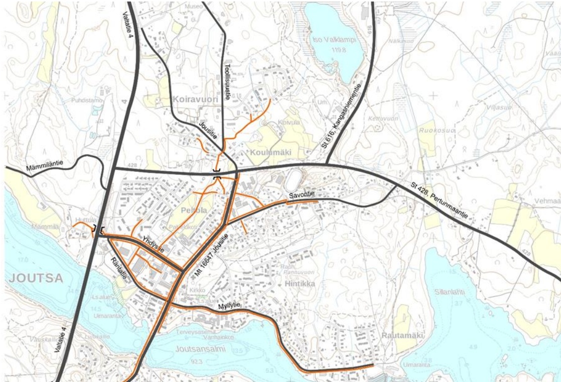
Kuva 9. Joutsan kirkonkylän kaava-alueita koskevat jalankulku- ja pyörätiet (oranssilla).
